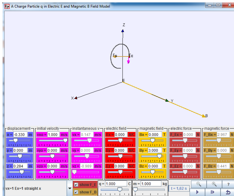
Figura 7: Movimento circular de uma carga imersa em um Campo Magnético. (Fonte: A pesquisa)
