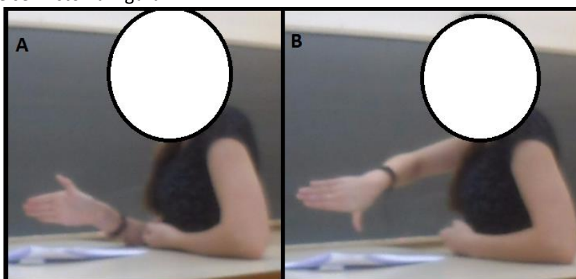
Figura 1: Gestos do aluno 1 indicando a regra da mão direita. (Fonte: A pesquisa)
