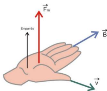
Figura 2: Regra da mão direita para a força magnética que atua em uma carga. (Fonte: https://www.todamateria.com.br/forca-magnetica/ )
