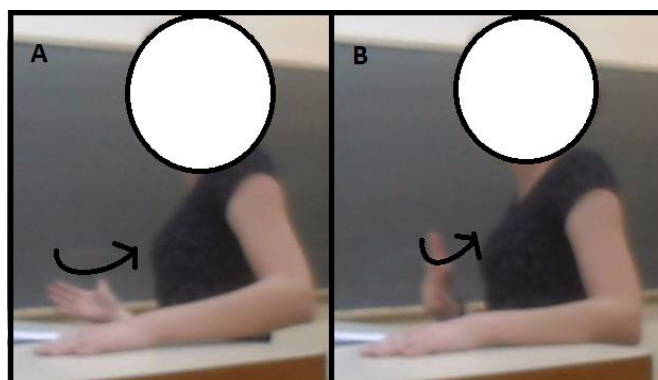
Figura 4: Movimento da mão de A1 demonstrando a força magnética resultante sobre a carga. (Fonte: A pesquisa)
