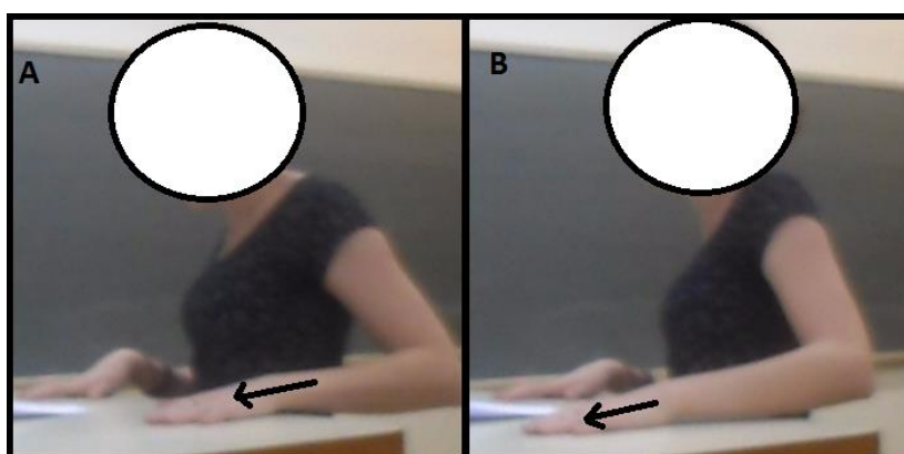
Figura 3: Movimento da mão de A1 demonstrando a Força Elétrica resultante sobre a carga. (Fonte: A pesquisa)
