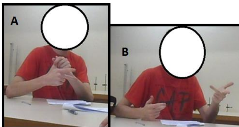
Figura 5: Aluno 2 (A2) explicando uma questão utilizando a regra da mão direita. (Fonte: A pesquisa)
