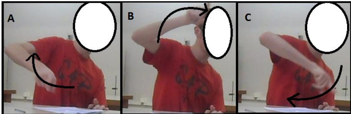
Figura 6: Movimento circular dinâmico de uma carga imersa em um campo magnético demonstrado pelo aluno 2. (Fonte: A pesquisa)
