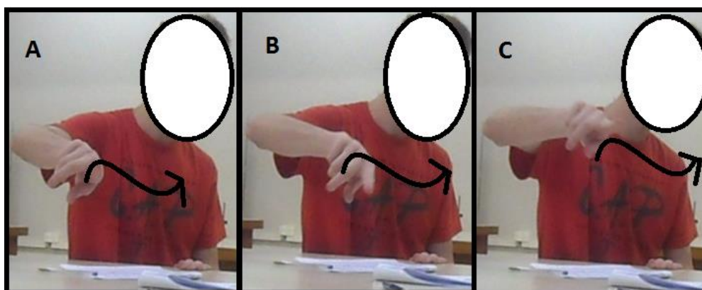
Figura 8: Movimento espiral dinâmico de uma carga imersa em um Campo Magnético apresentado pelo aluno 2. (Fonte: A pesquisa)
